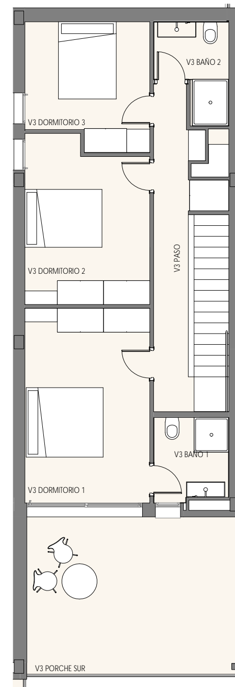
PLANTA PRIMERA
